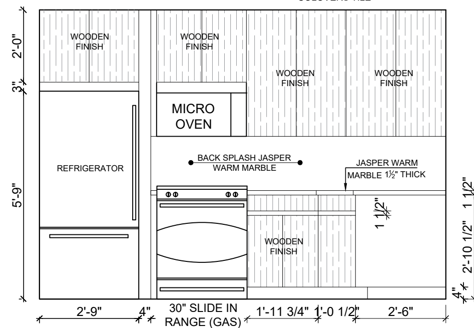
ELEVATION-A
